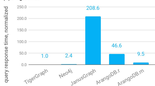
(B) PageRank
